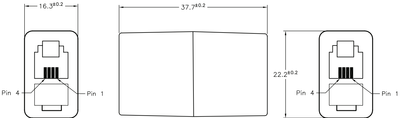
Dimensions : Millimetres
