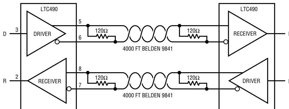
LTC490 • TA01
