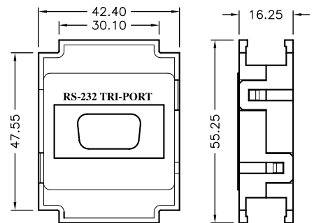
Dimensions : Millimeters (Inchs)
