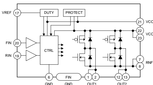
Fig.5 BD6212FP
