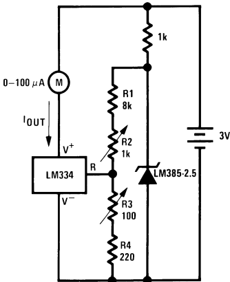
0°C–100°C Thermometer
