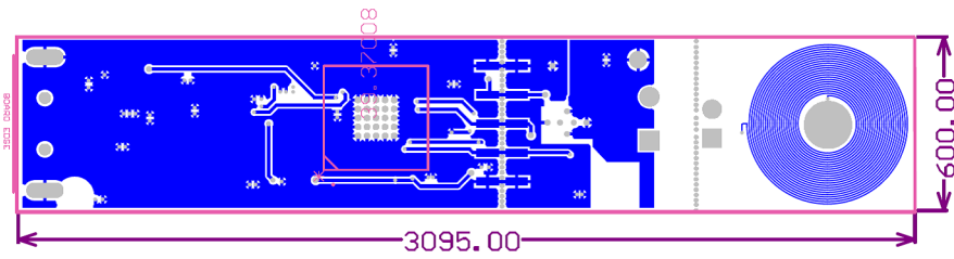
Figure 4-3. Bottom Layer
