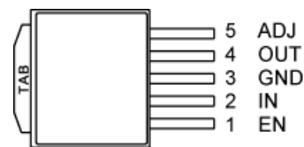
5-Pin TO-252 (D-Pak) Adjustable Voltage (D) MIC29152
