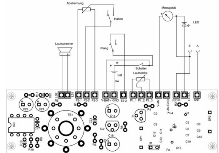
Der Verdrahtungsplan
