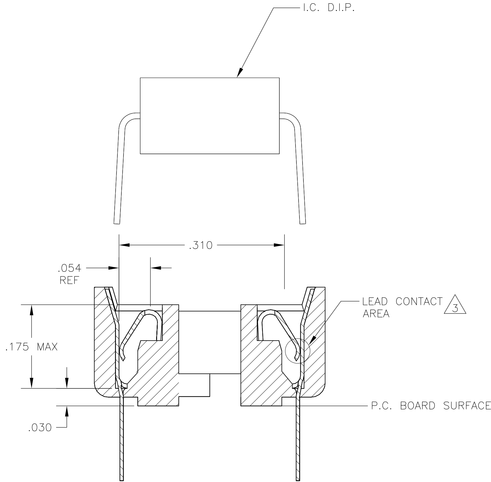
SECTION A-A SCALE 10:1
