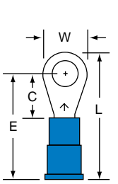
MV14-10R/L Stud Size 10 Wire Range 16-14
