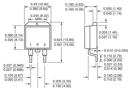
TO-263AB
